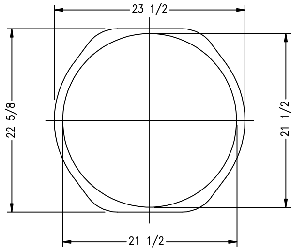
BOTTOM FLANGE
