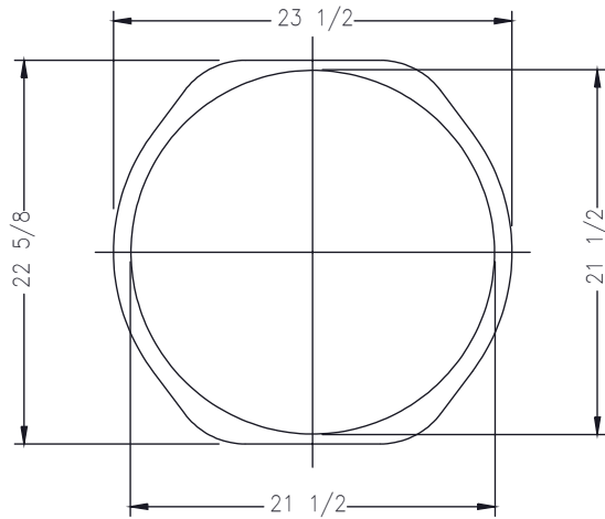
BOTTOM FLANGE
