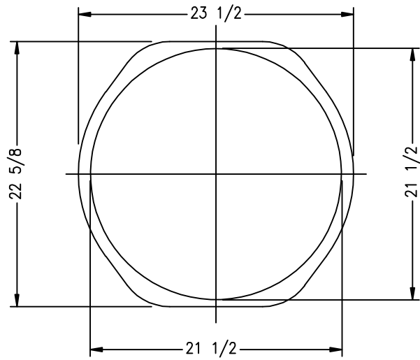
BOTTOM FLANGE
